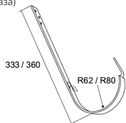
Крюк длинный (125/150) толщина стали: 1,0 мм (сталь 1,0 мм свёрнута 4 раза)
