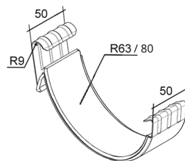
Соединитель желоба (125/150) толщина стали: 1,0 мм
