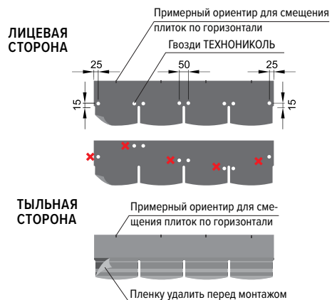
Рис. 4. Схема крепления фасадной плитки на 8 гвоздей
