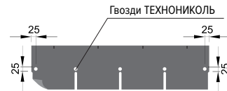
Рис. 5. Схема крепления фасадной плитки на 5 гвоздей
