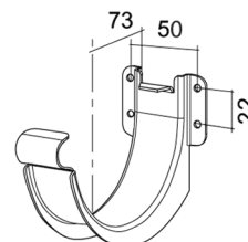
Крюк короткий (125) толщина стали: 1,0 мм
